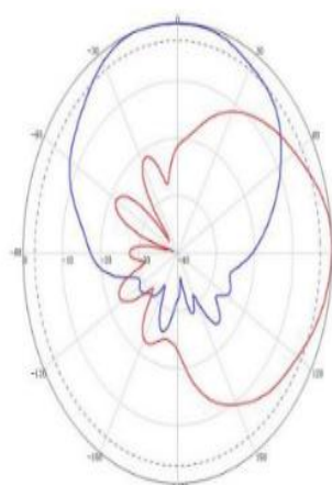
1710 ~ 2700MHz: ±45° Pol.
