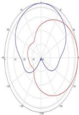
698 ~ 960MHz: ±45° Pol.
